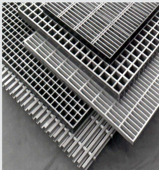
NẠP MƯƠNG GRATING
